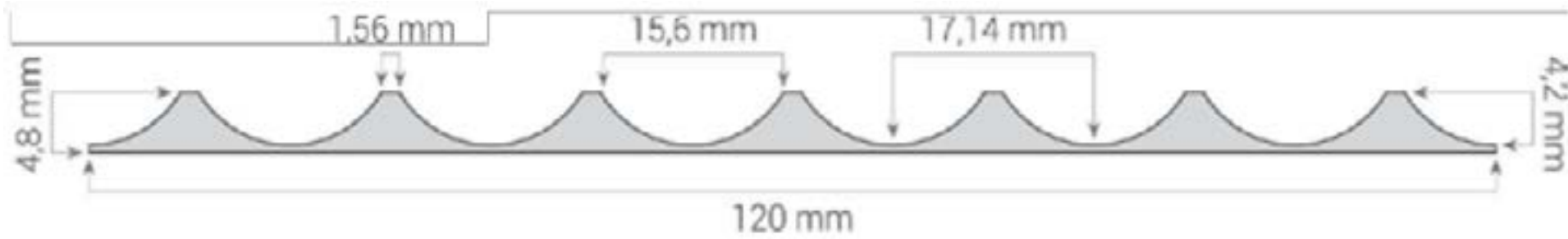
Desenho técnico (secção 120 mm):
